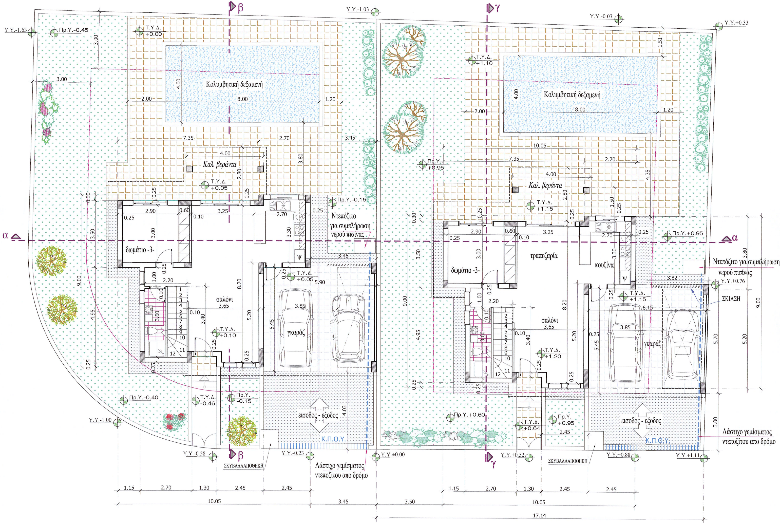
Κάτοψη ισογείου.
